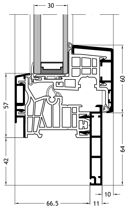
Telaio a Z D2X con anta Nova-line A10
