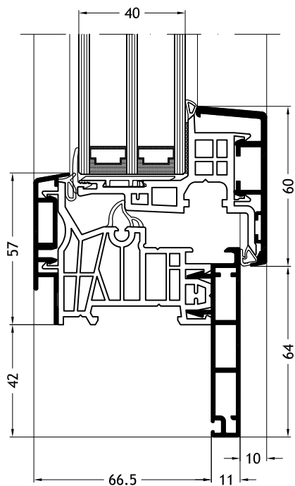
Telaio a Z D2X con anta Nova-line A11
